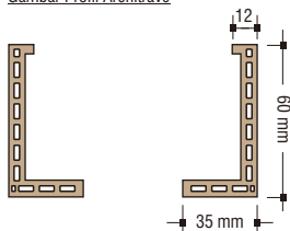
Gambar Profil Architrave
