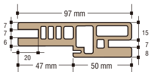
Gambar Profil Kusen
