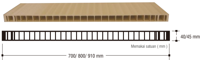
Gambar Profil Pintu
