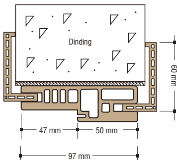
Ilustrasi Pemasangan Kusen + Architrave
